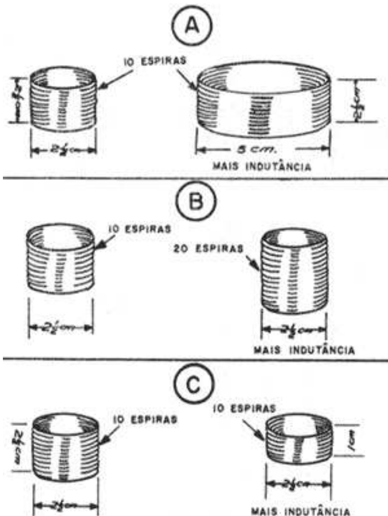
Figura 3.2: Propriedades da indutância
