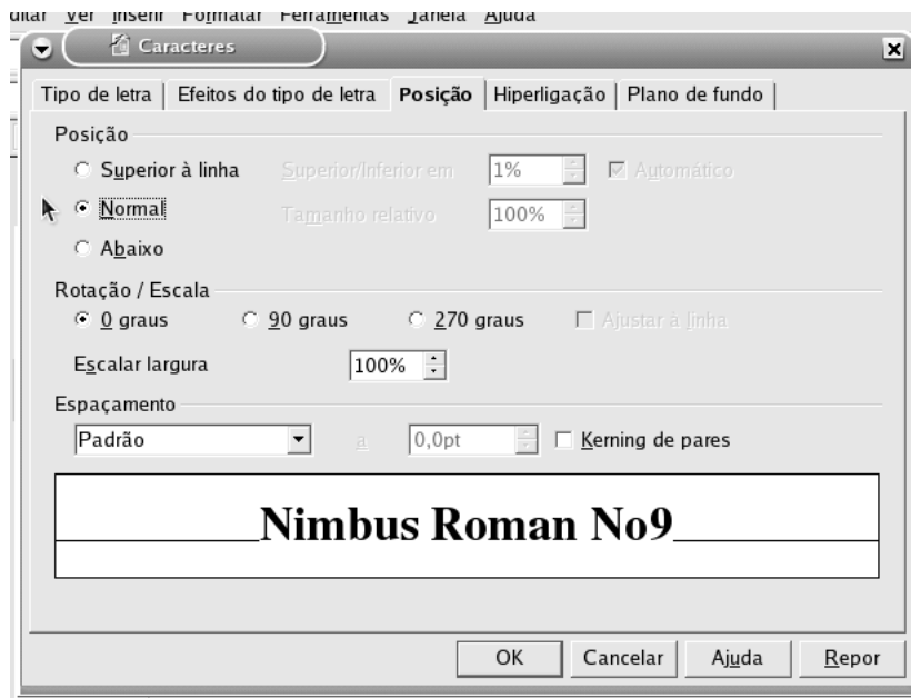
Figura 18.14: Aba “Posição”
