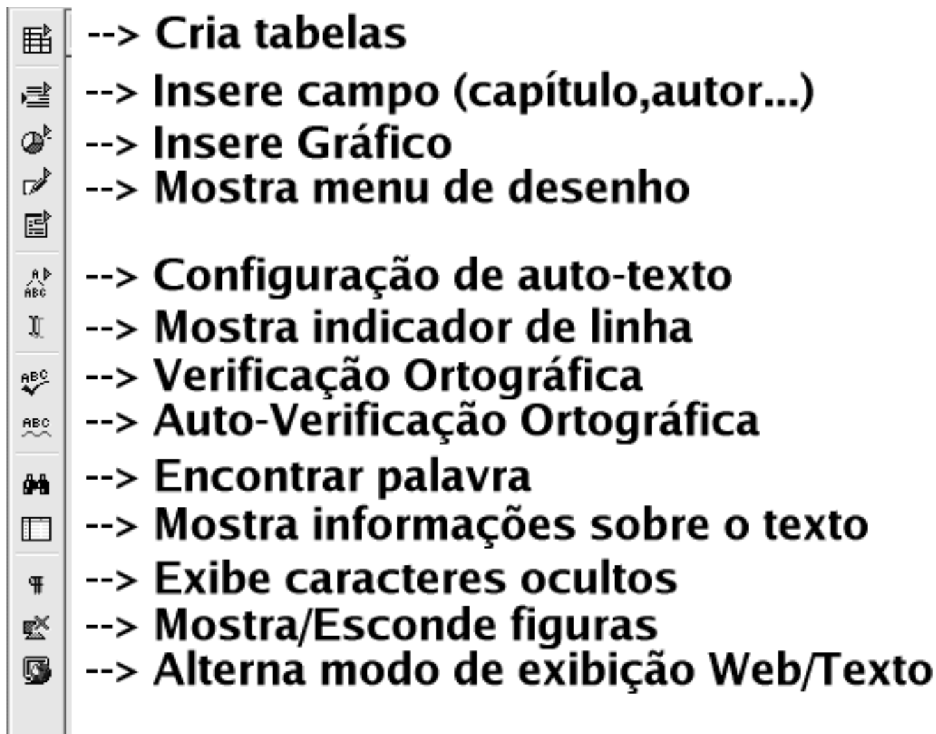
Figura 18.4: Barra lateral
